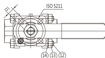
材質表:
